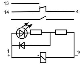
РПГ-16-101-60 с индикатором и помехоподавляющими элементами
