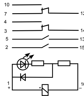
РПГ-16-202-60 с индикатором и помехоподавляющими элементами
