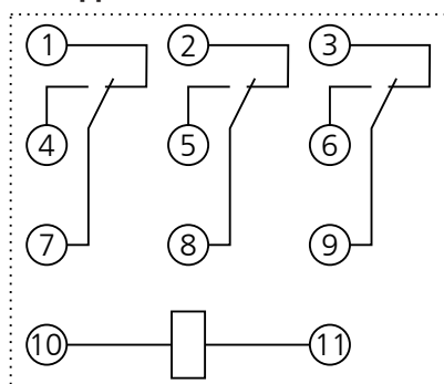
Реле РП-63 с 3-мя переключающими контактами
