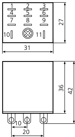
Реле РП-63 с 3-мя переключающими контактами
