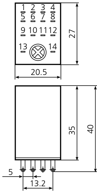
Реле РЭК 78/4 с 4-мя переключающими контактами
