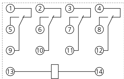
Реле РЭК 78/4 с 4-мя переключающими контактами
