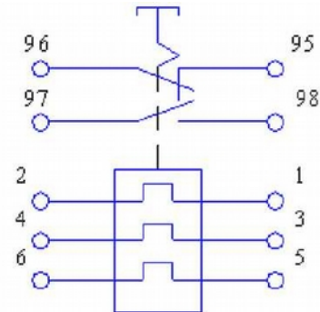
б) Реле с размыкающим и замыкающим контактами
