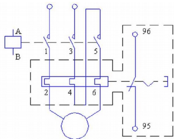
б) в цепь двухфазной нагрузки и в цепь постоянного тока
