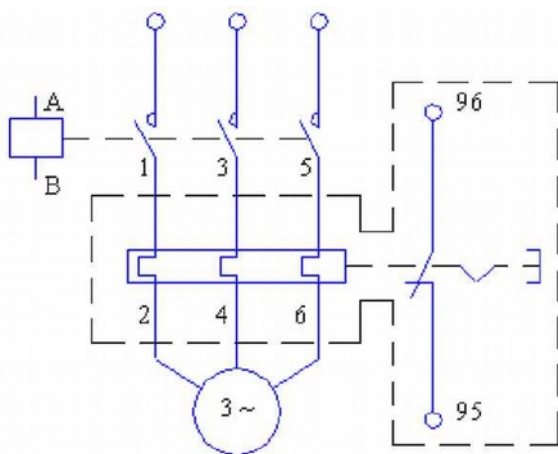
а) в цепь трехфазной нагрузки;
