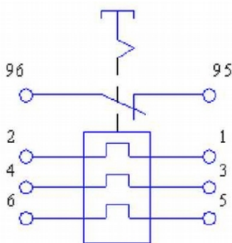
а) Реле с размыкающим контактом
