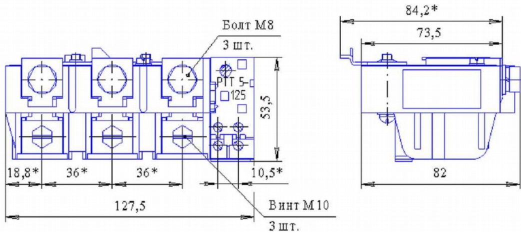
Рис. 5.7 - Исполнение реле для подсоединения к пускателю
