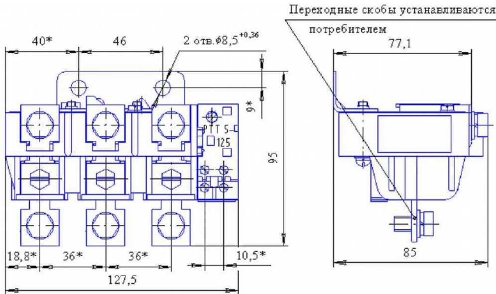
Рис. 5.10 - Исполнение реле для индивидуальной установки с подсоединением внешних проводов при помощи кабельных наконечников
