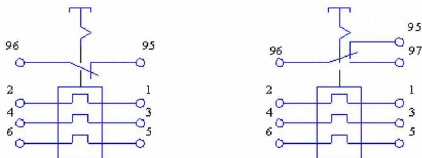
а) с размыкающим контактом б) с переключающим контактом
