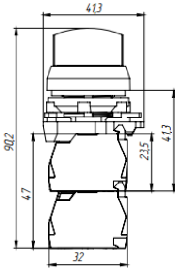
Рис.2. Переключатель управления с рукояткой.
