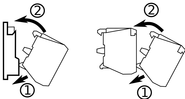
Рис.1. Монтаж и демонтаж блоков контактов.
