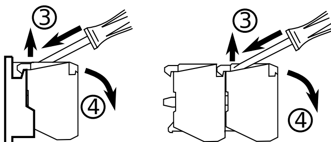
Рис.1. Монтаж и демонтаж блоков контактов.
